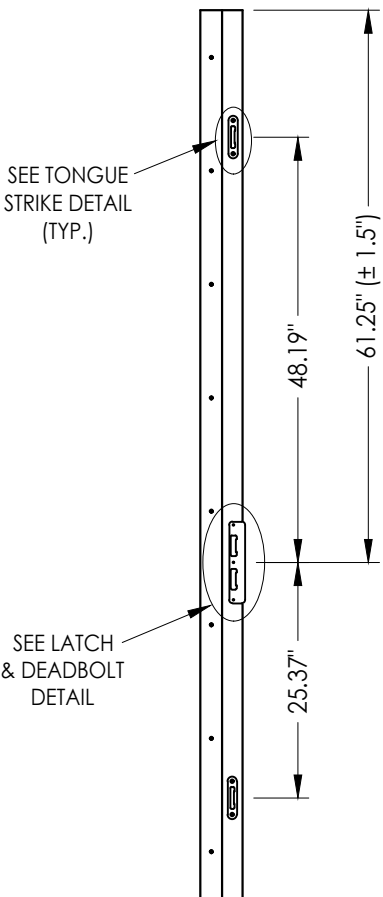
STRIKE JAMB
