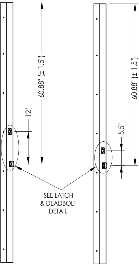
STRIKE JAMB
